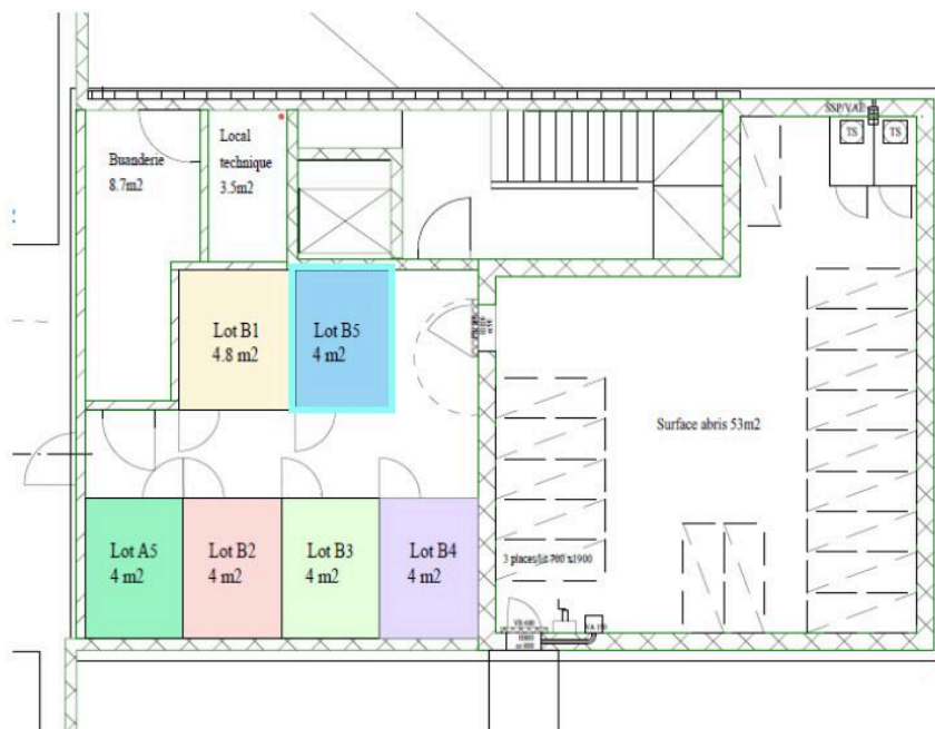
Sous-sol, bâtiment Est – caves et abri PC
